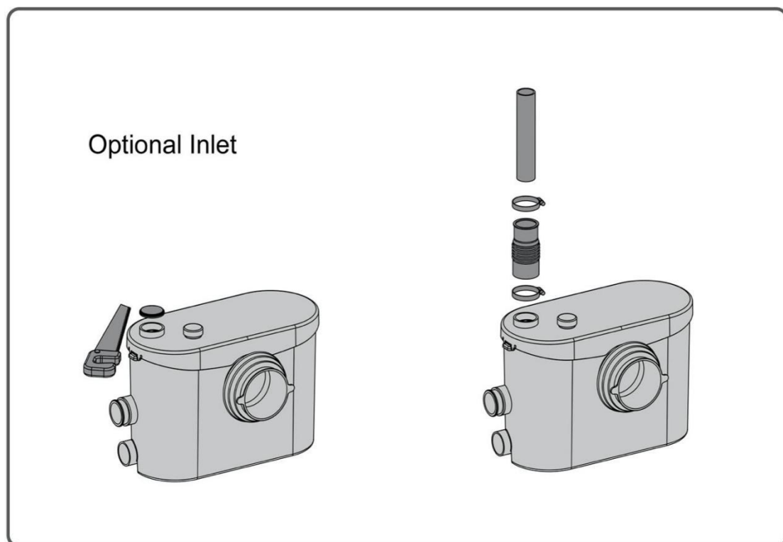
Fig 8: Optional top inlet
