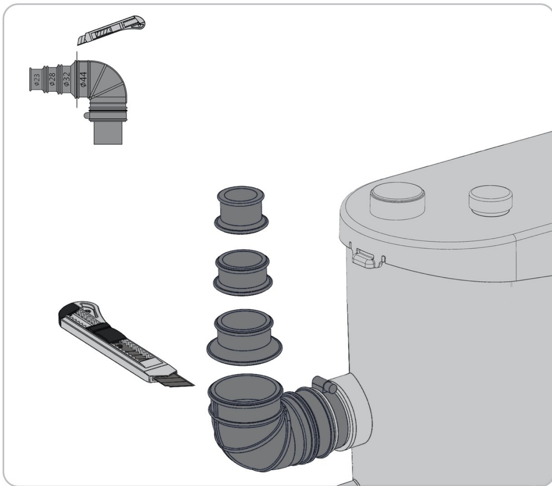
Fig 8: Optional top inlet
